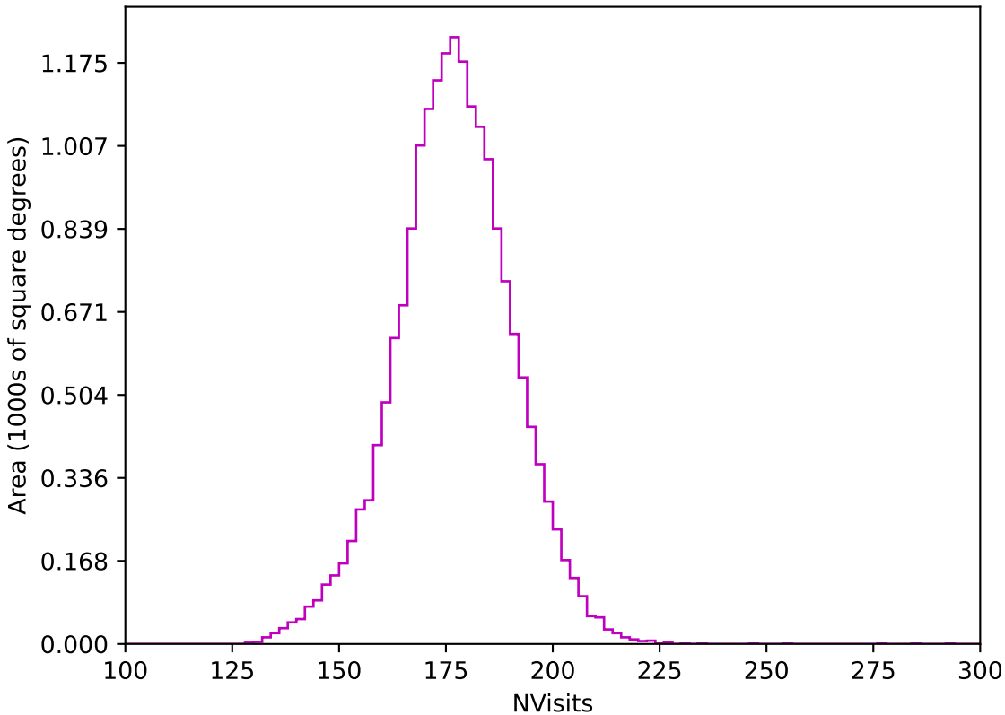
weather_cloudso35v3.4_10yrs WFD z band: NVisits
