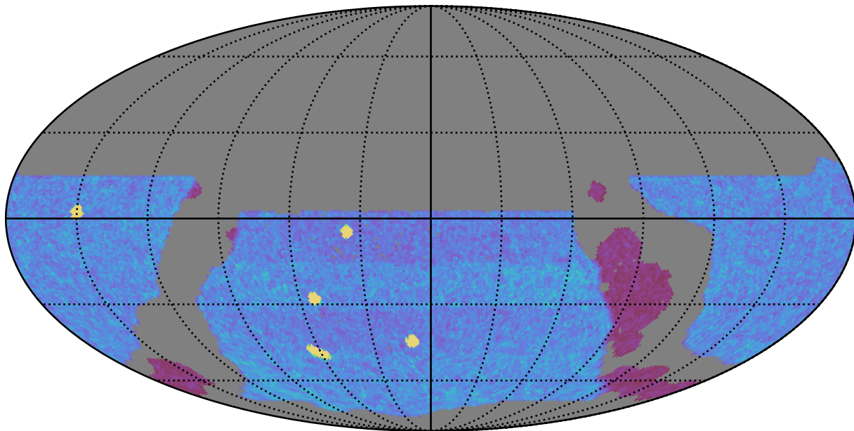
weather_cloudso35v3.4_10yrs WFD y band: NVisits
