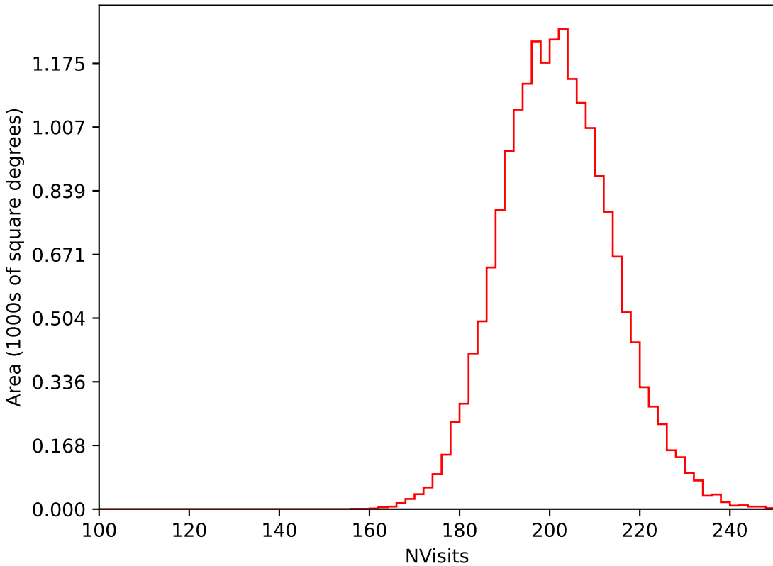
weather_cloudso35v3.4_10yrs WFD i band: NVisits
