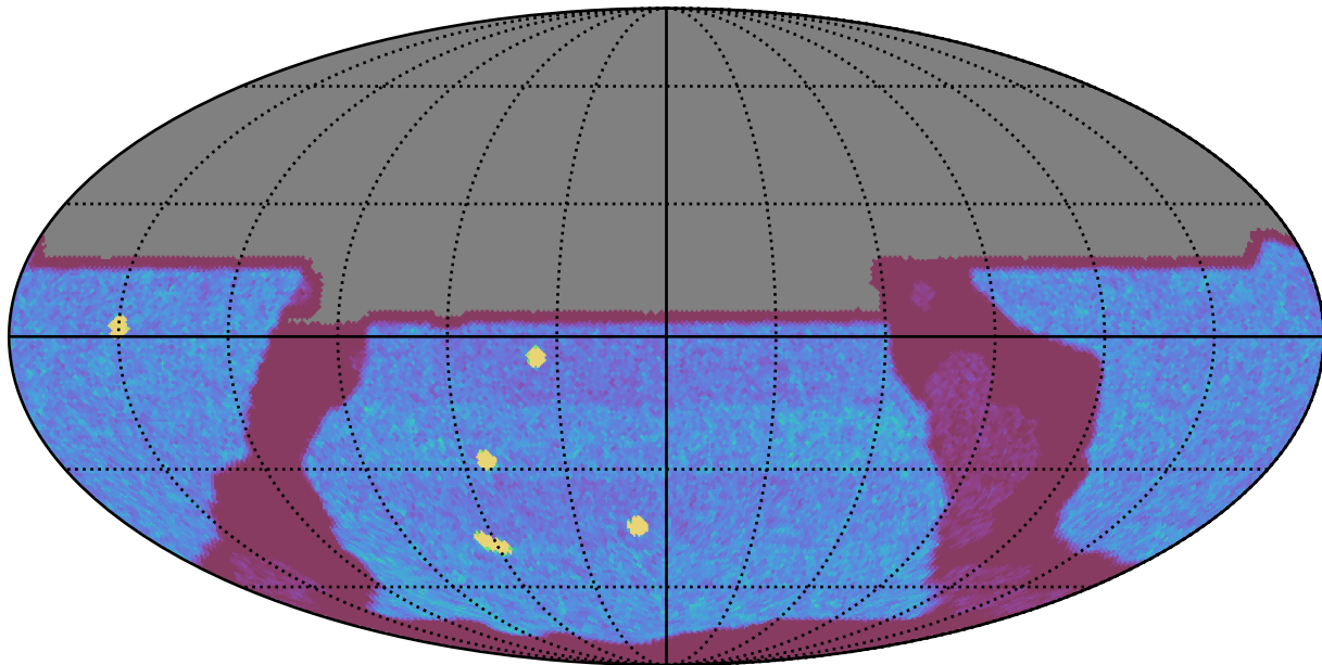
weather_cloudso35v3.4_10yrs All sky y band: NVisits
