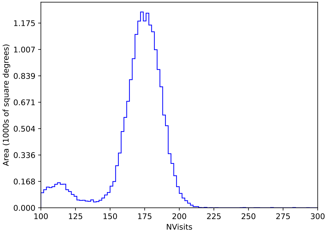
weather_cloudso35v3.4_10yrs All sky y band: NVisits
