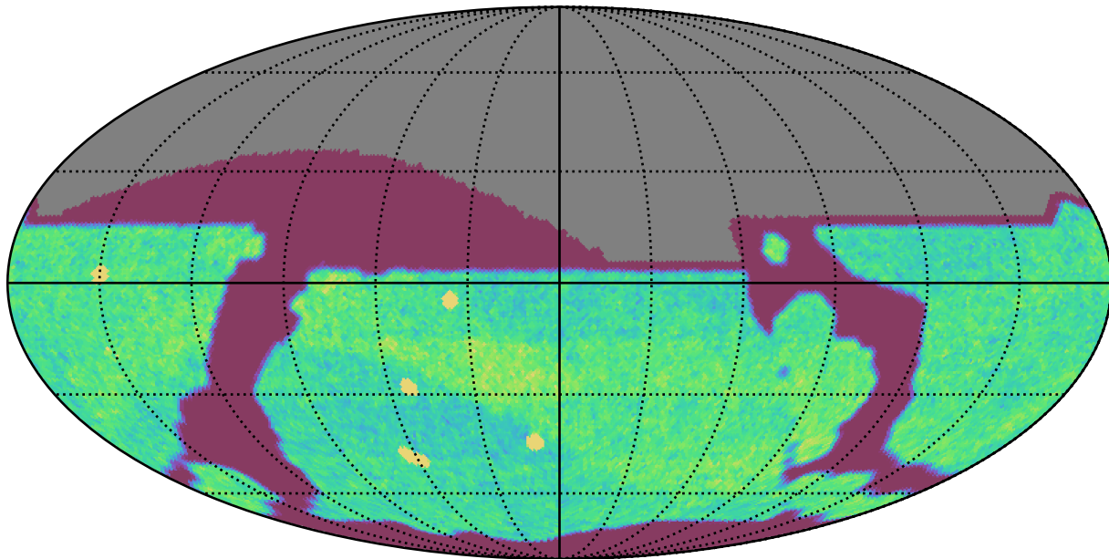
weather_cloudso35v3.4_10yrs All sky i band: NVisits
