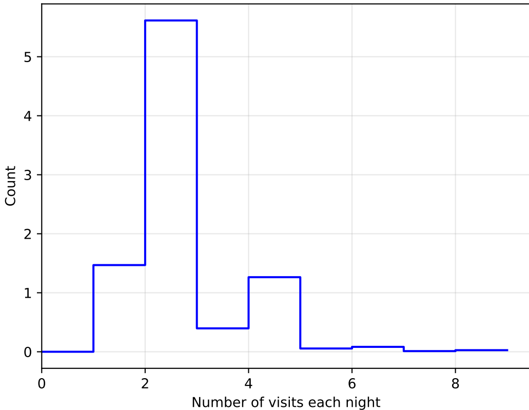
1e6 weather_cloudso35v3.4_10yrs WFD: NVisitsPerNight
