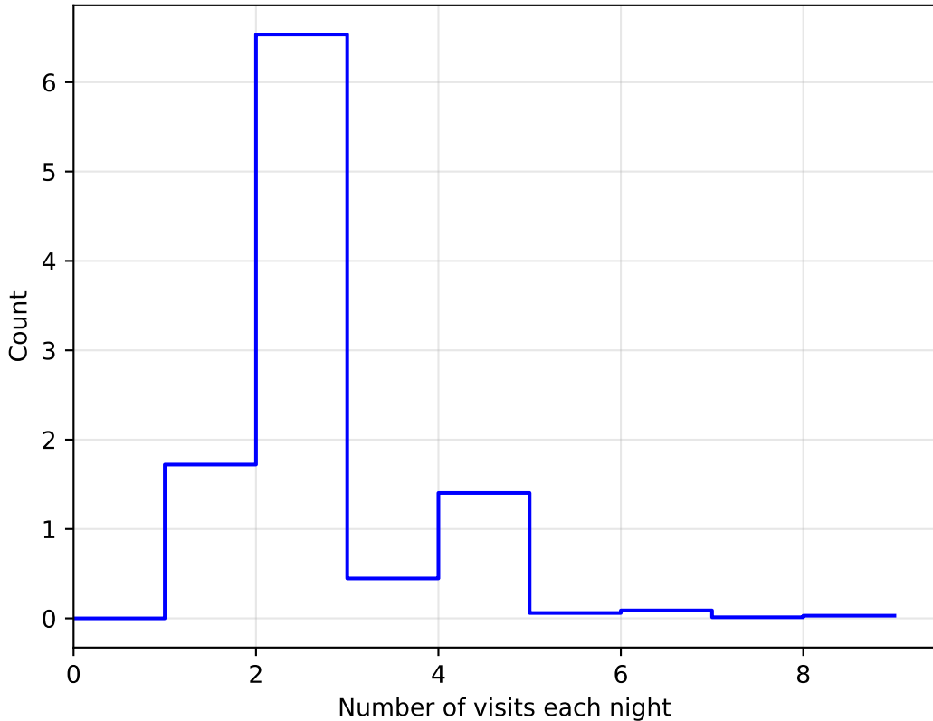
weather_cloudso35v3.4_10yrs All sky: NVisitsPerNight
