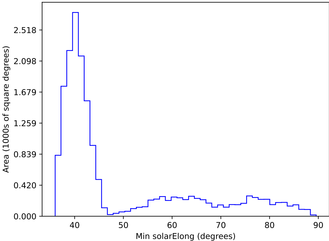
weather_cloudso35v3.4_10yrs WFD z band: Min solarElong
