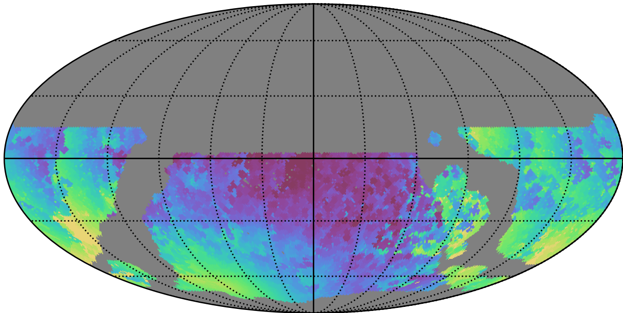
weather_cloudso35v3.4_10yrs WFD y band: Min solarElong
