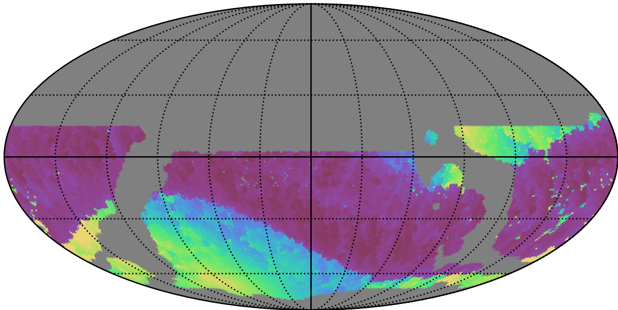
weather_cloudso35v3.4_10yrs WFD i band: Min solarElong
