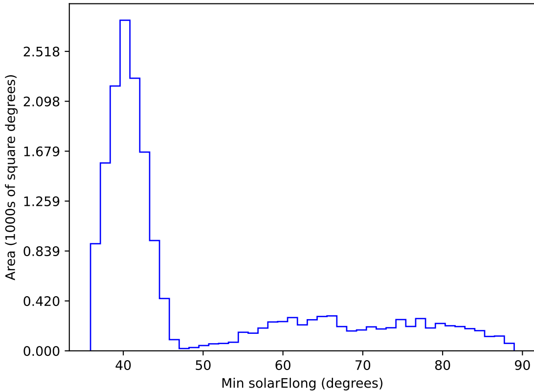
weather_cloudso35v3.4_10yrs WFD i band: Min solarElong
