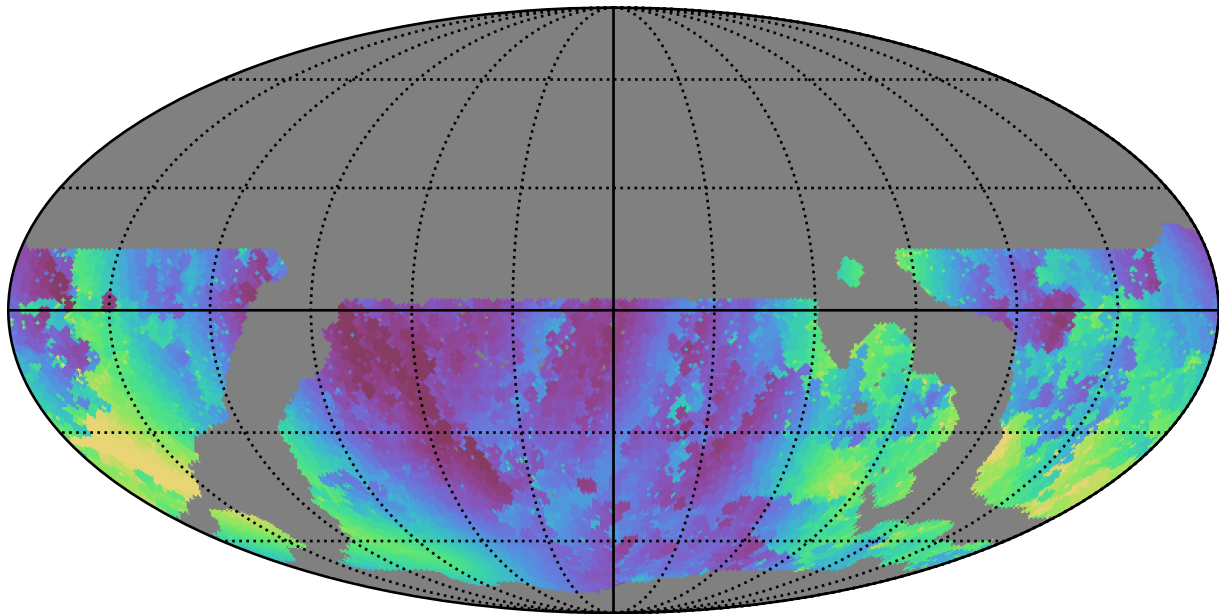
weather_cloudso35v3.4_10yrs WFD g band: Min solarElong
