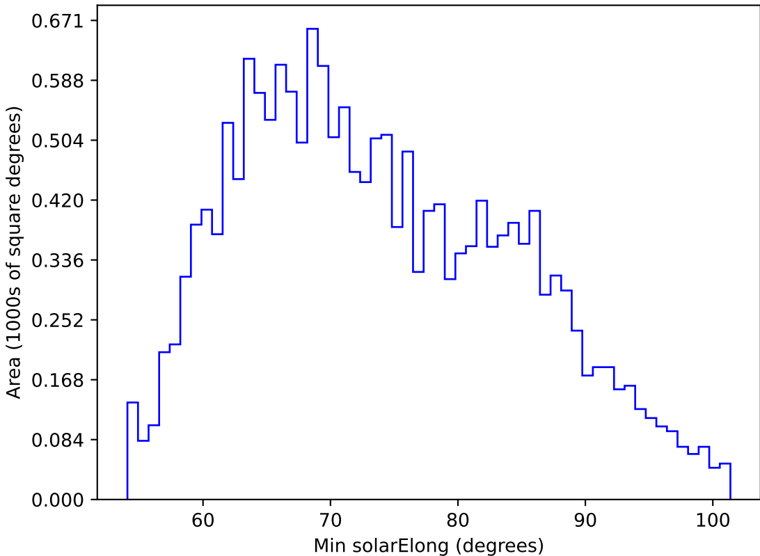
weather_cloudso35v3.4_10yrs WFD g band: Min solarElong
