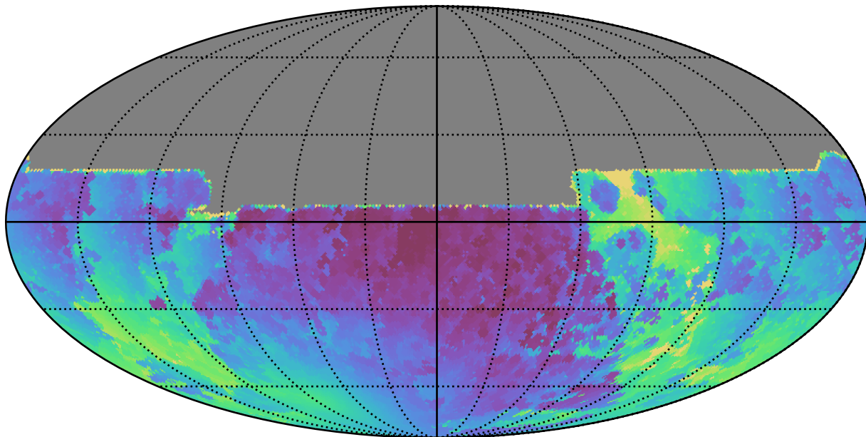
weather_cloudso35v3.4_10yrs All sky y band: Min solarElong
