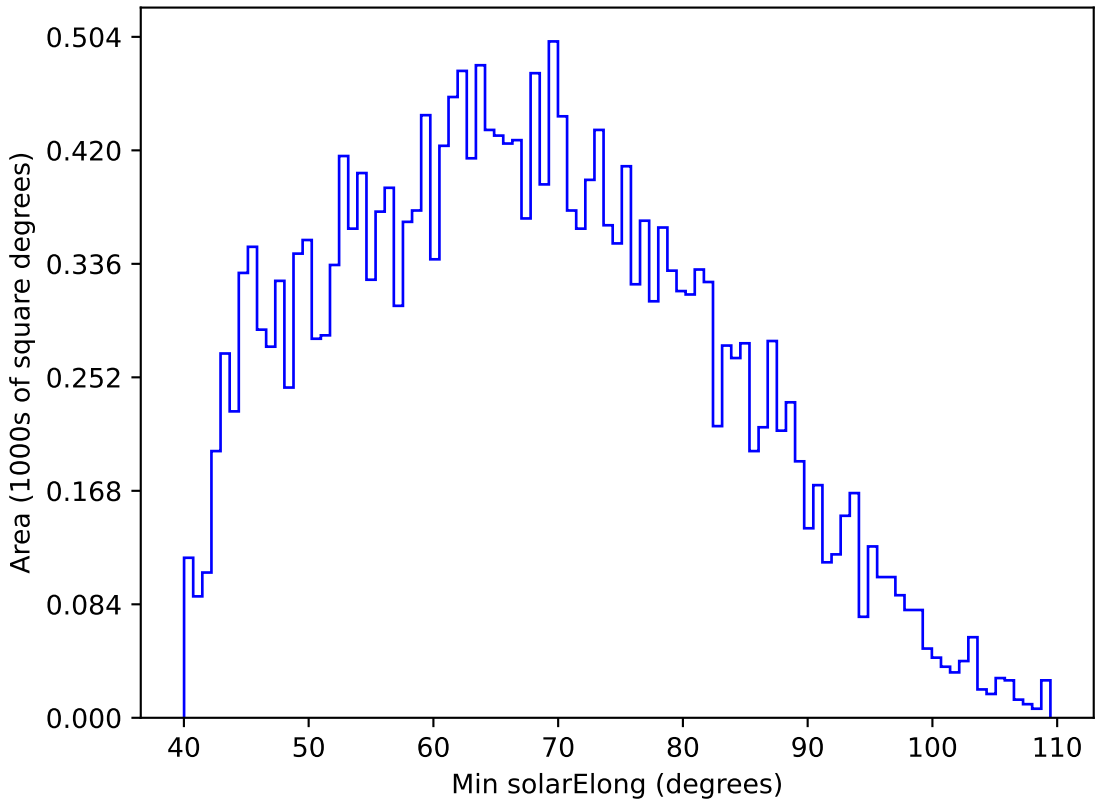
weather_cloudso35v3.4_10yrs All sky y band: Min solarElong
