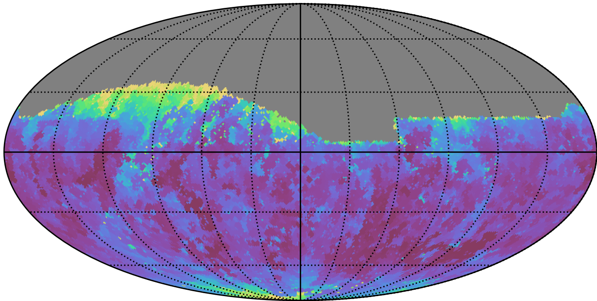
weather_cloudso35v3.4_10yrs Yr 1 z band: Min seeingGeom
