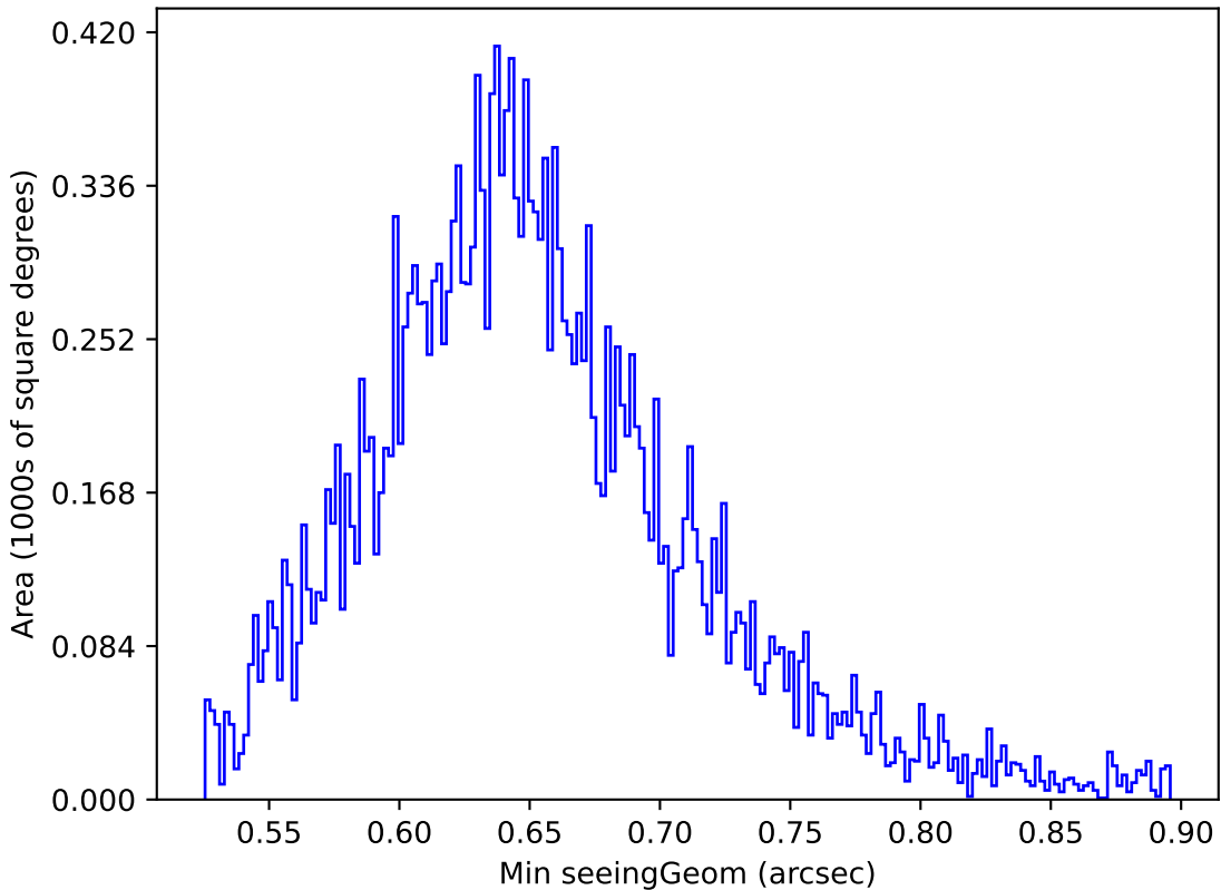
weather_cloudso35v3.4_10yrs Yr 1 y band: Min seeingGeom
