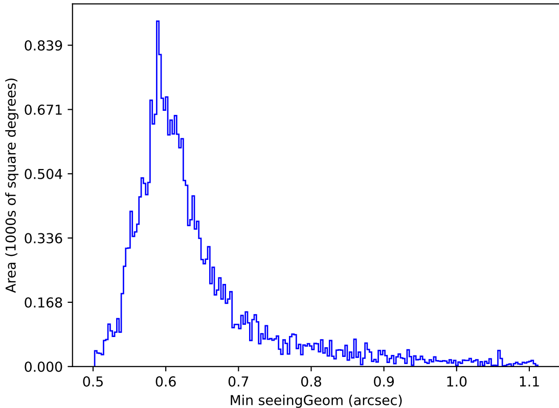
weather_cloudso35v3.4_10yrs Yr 1 i band: Min seeingGeom
