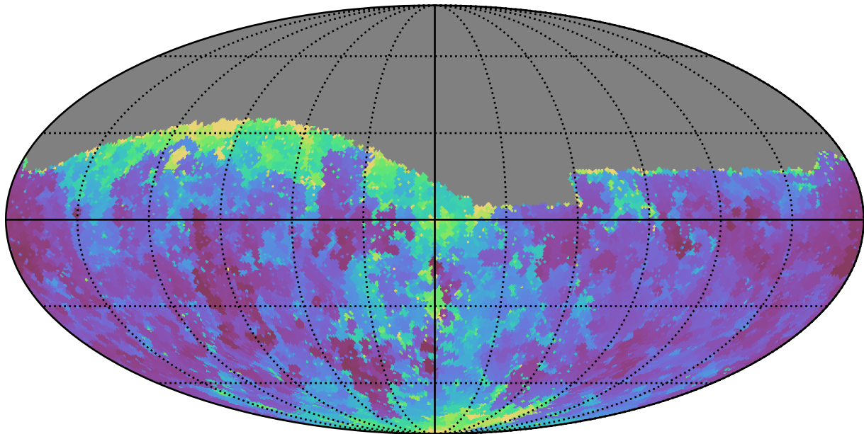
weather_cloudso35v3.4_10yrs Yr 1 g band: Min seeingGeom
