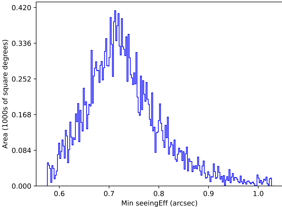
weather_cloudso35v3.4_10yrs Yr 1 y band: Min seeingEff
