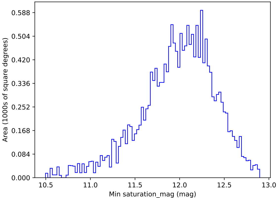
weather_cloudso35v3.4_10yrs WFD z band: Min saturation_mag
