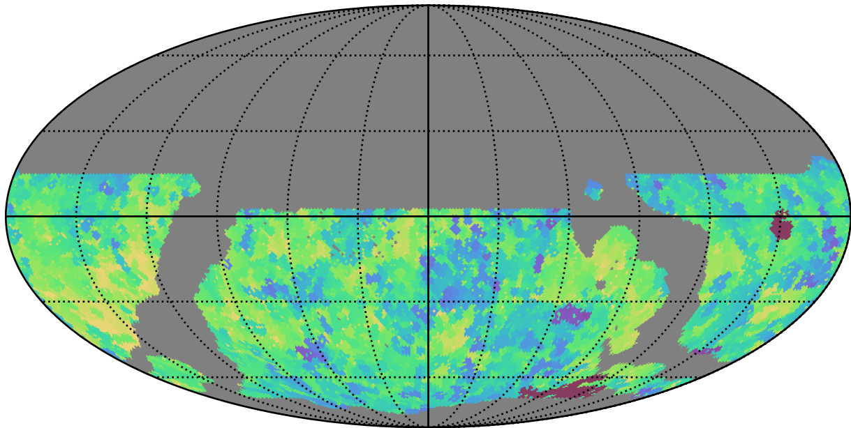
weather_cloudso35v3.4_10yrs WFD y band: Min saturation_mag
