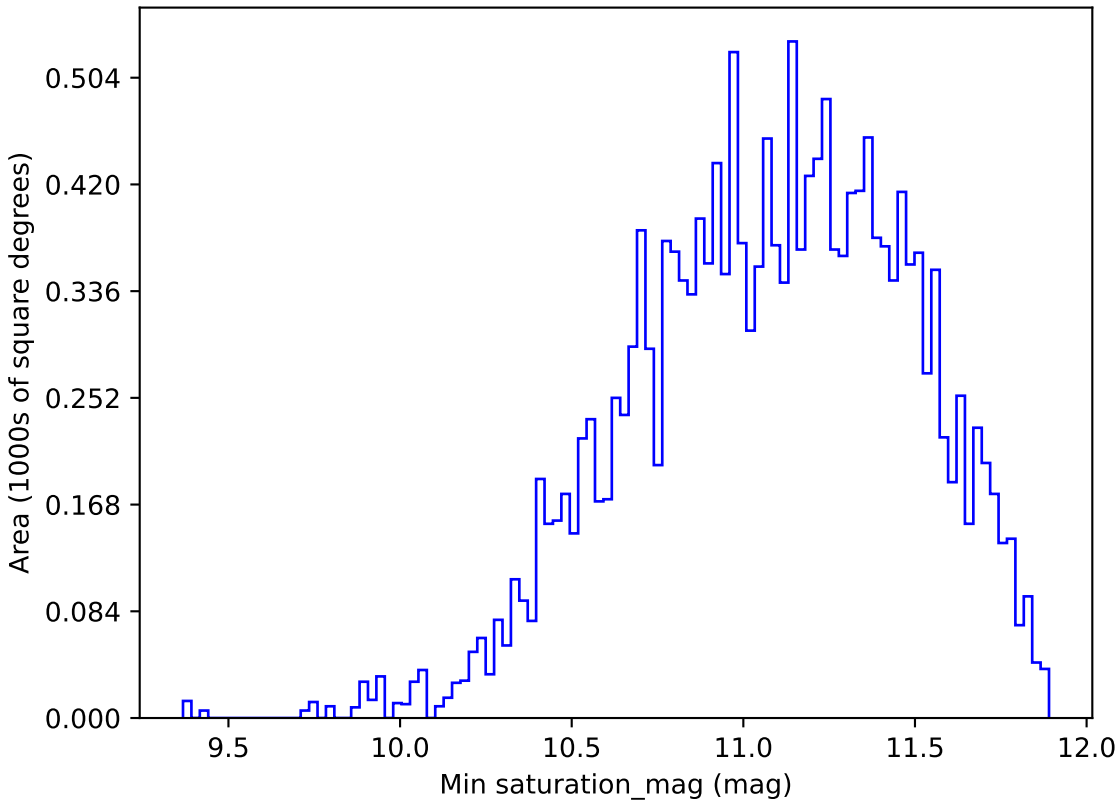
weather_cloudso35v3.4_10yrs WFD y band: Min saturation_mag
