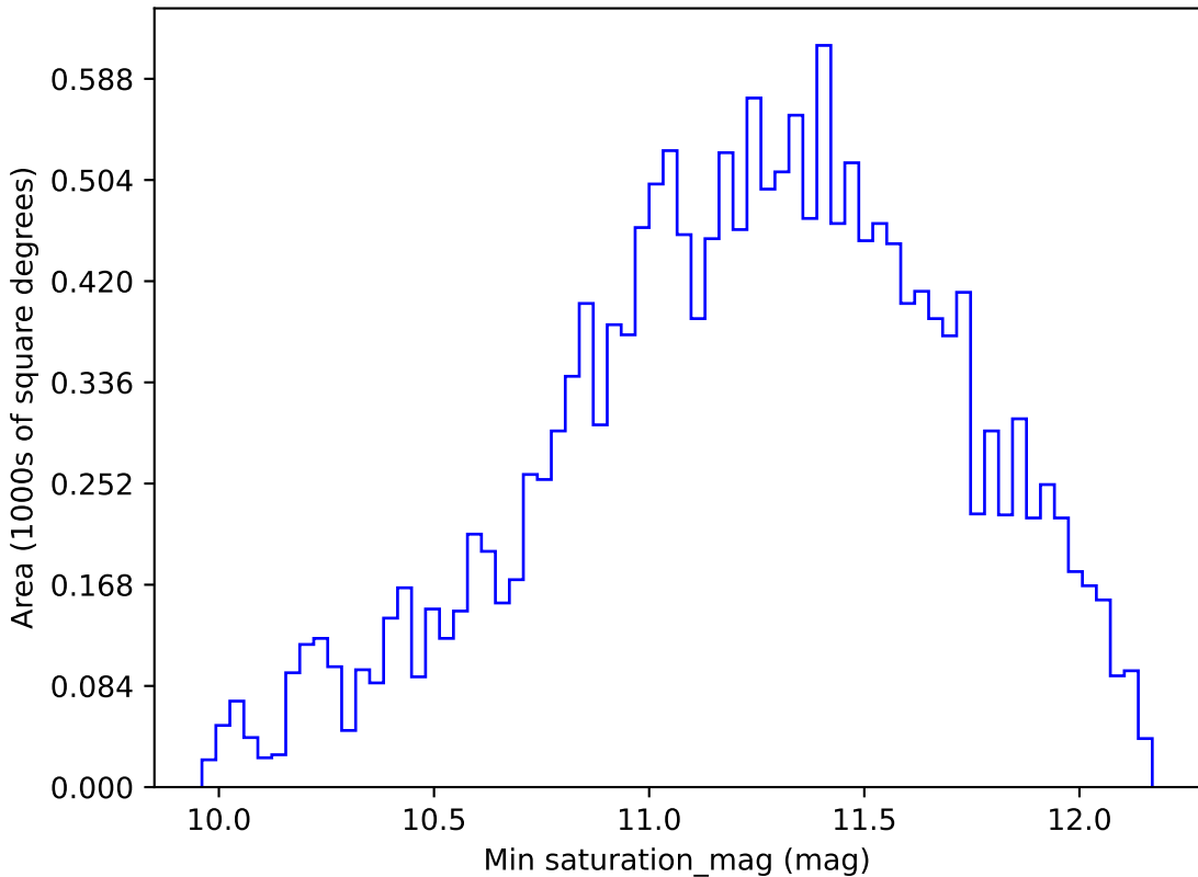
weather_cloudso35v3.4_10yrs WFD u band: Min saturation_mag
