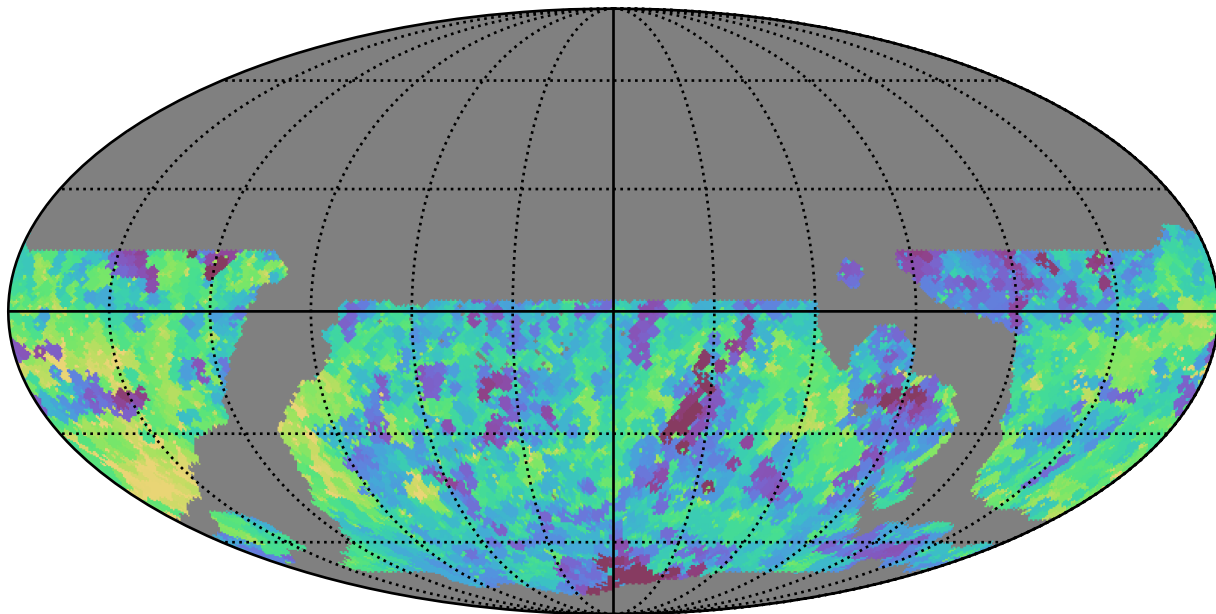
weather_cloudso35v3.4_10yrs WFD r band: Min saturation_mag
