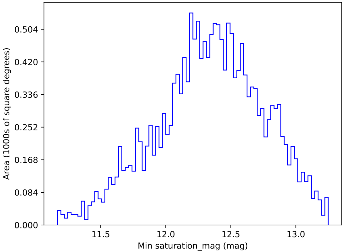
weather_cloudso35v3.4_10yrs WFD r band: Min saturation_mag
