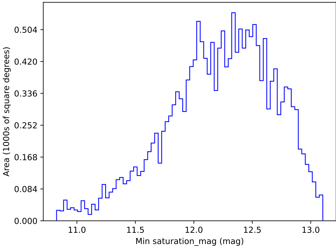
weather_cloudso35v3.4_10yrs WFD i band: Min saturation_mag
