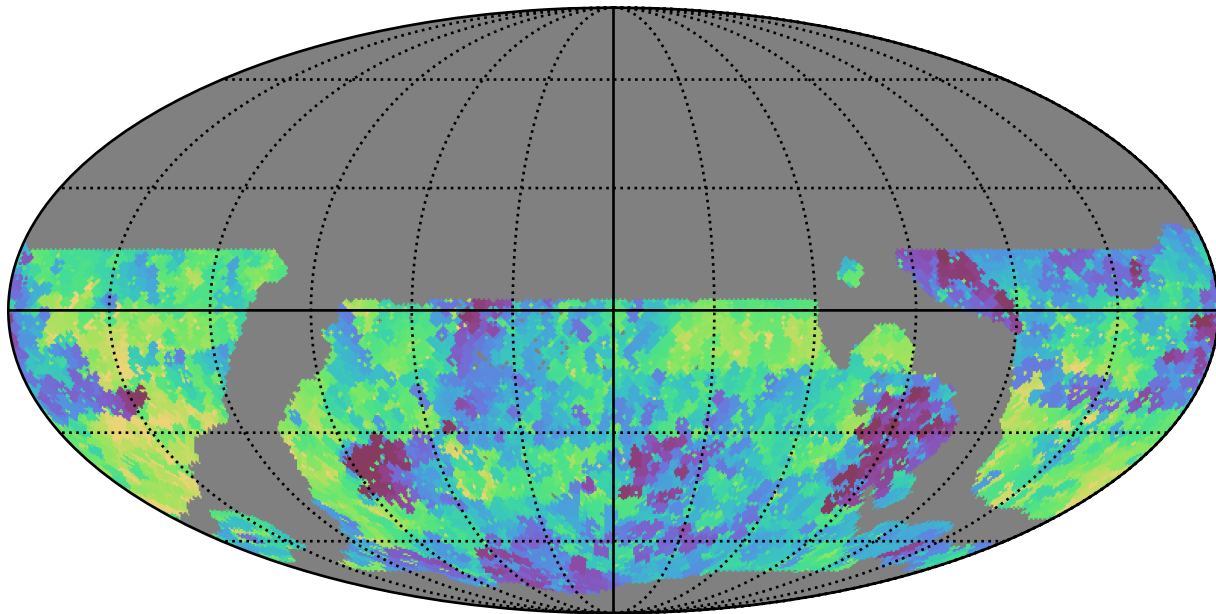
weather_cloudso35v3.4_10yrs WFD g band: Min saturation_mag
