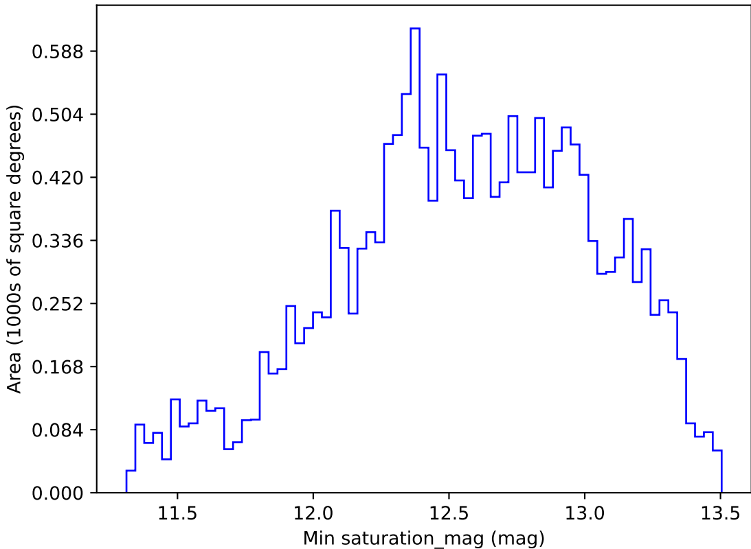
weather_cloudso35v3.4_10yrs WFD g band: Min saturation_mag
