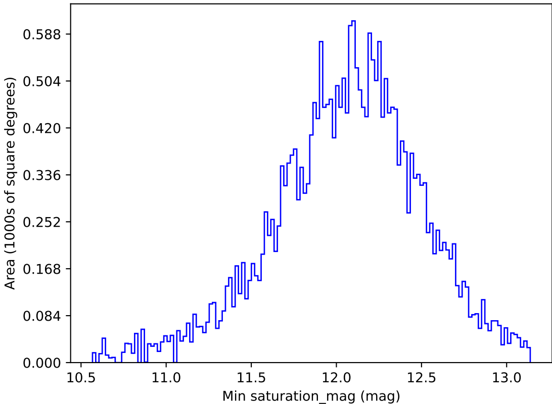
weather_cloudso35v3.4_10yrs All sky z band: Min saturation_mag
