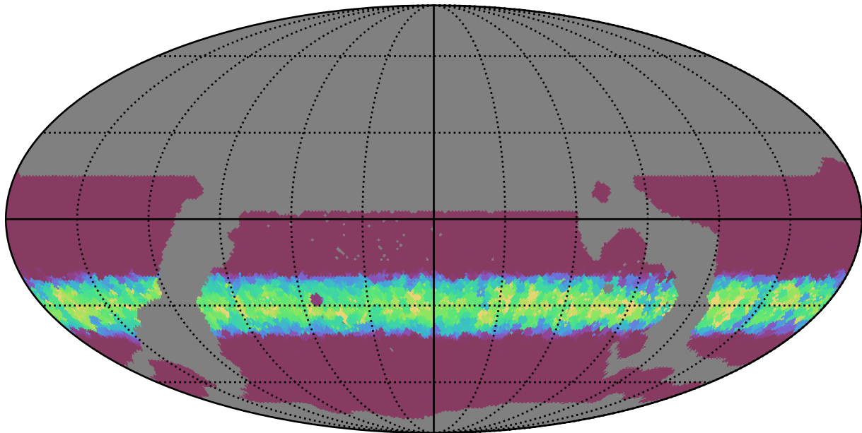
weather_cloudso35v3.4_10yrs WFD z band: Min normairmass
