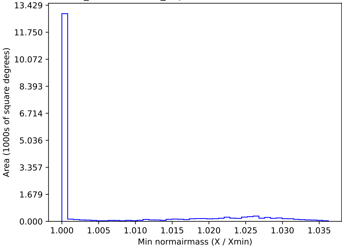
weather_cloudso35v3.4_10yrs WFD z band: Min normairmass
