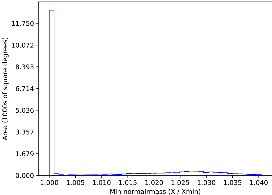
weather_cloudso35v3.4_10yrs WFD y band: Min normairmass
