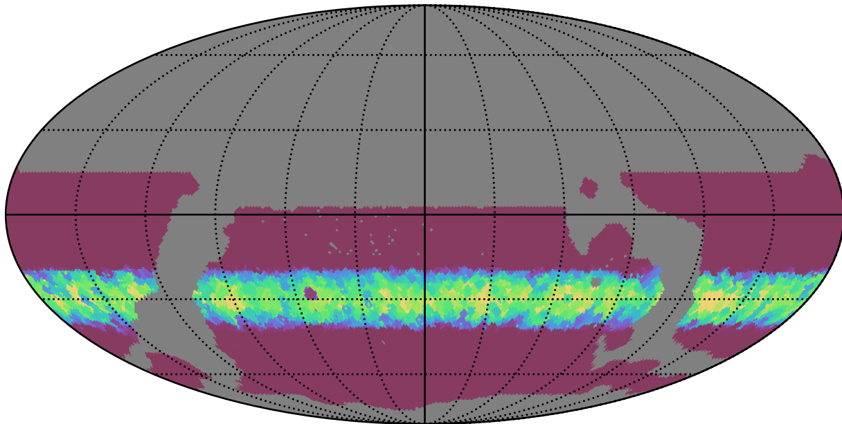
weather_cloudso35v3.4_10yrs WFD i band: Min normairmass
