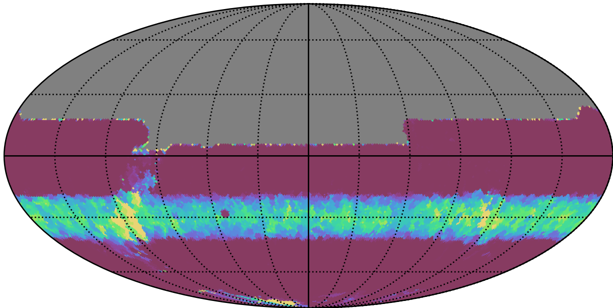
weather_cloudso35v3.4_10yrs All sky y band: Min normairmass
