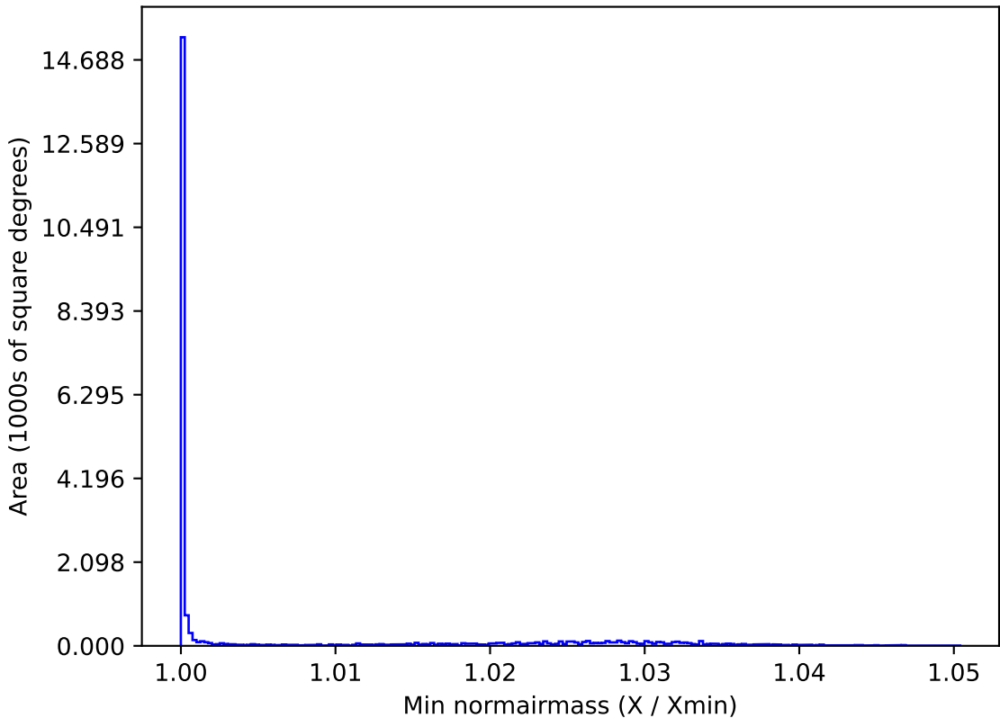
weather_cloudso35v3.4_10yrs All sky y band: Min normairmass
