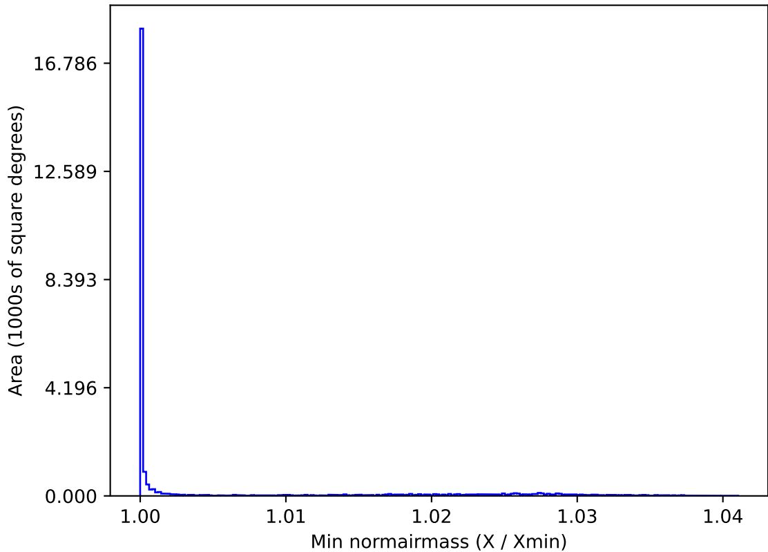
weather_cloudso35v3.4_10yrs All sky i band: Min normairmass
