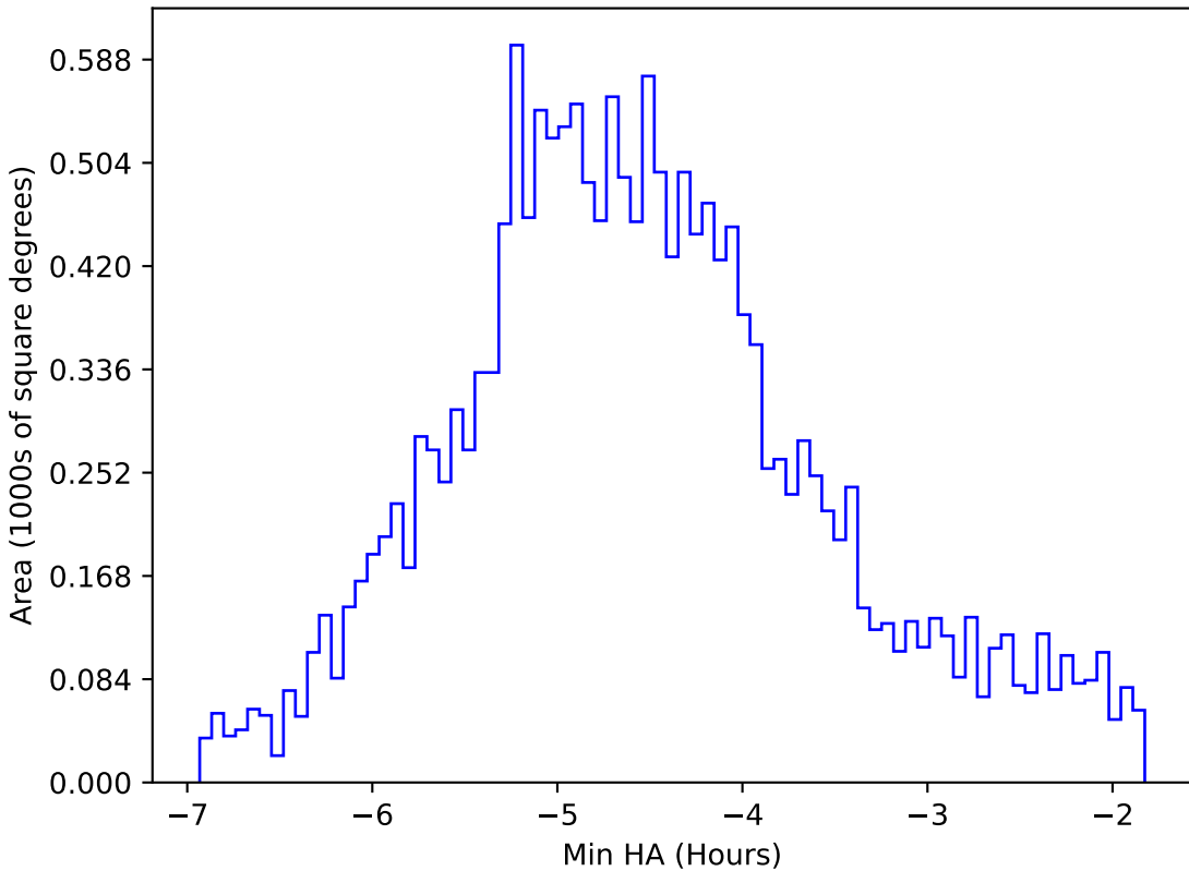
weather_cloudso35v3.4_10yrs WFD z band: Min HA
