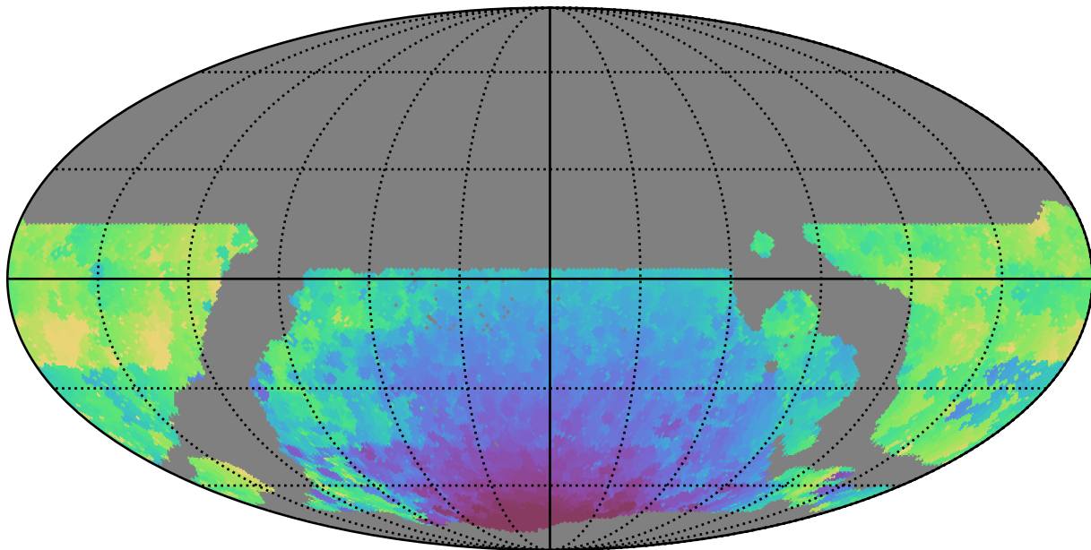
weather_cloudso35v3.4_10yrs WFD y band: Min HA
