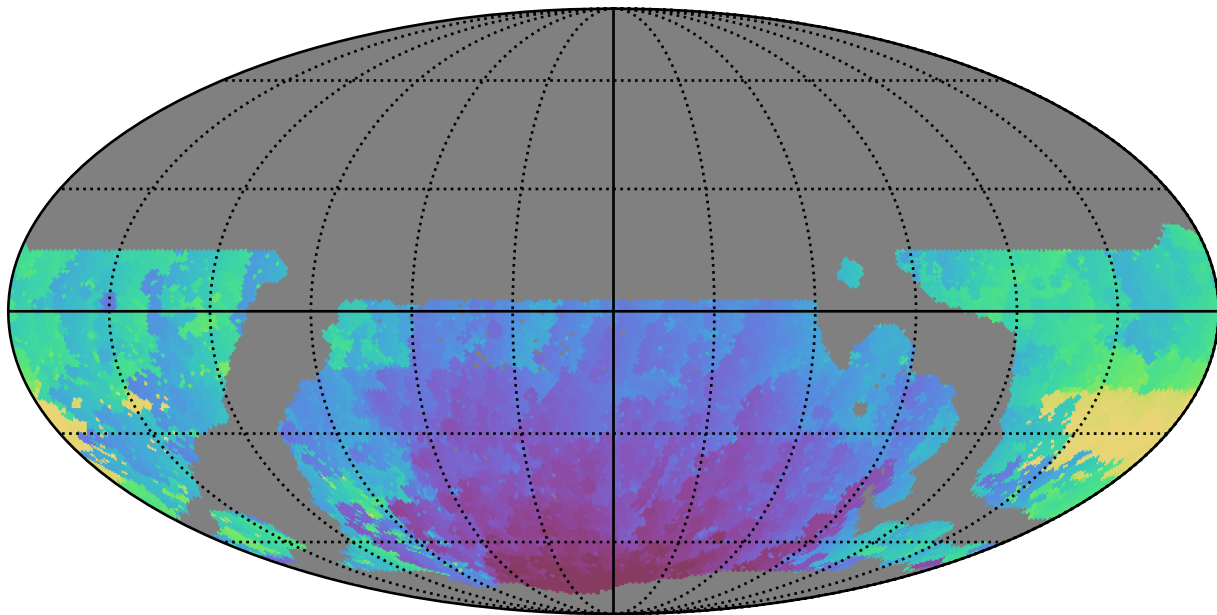
weather_cloudso35v3.4_10yrs WFD u band: Min HA
