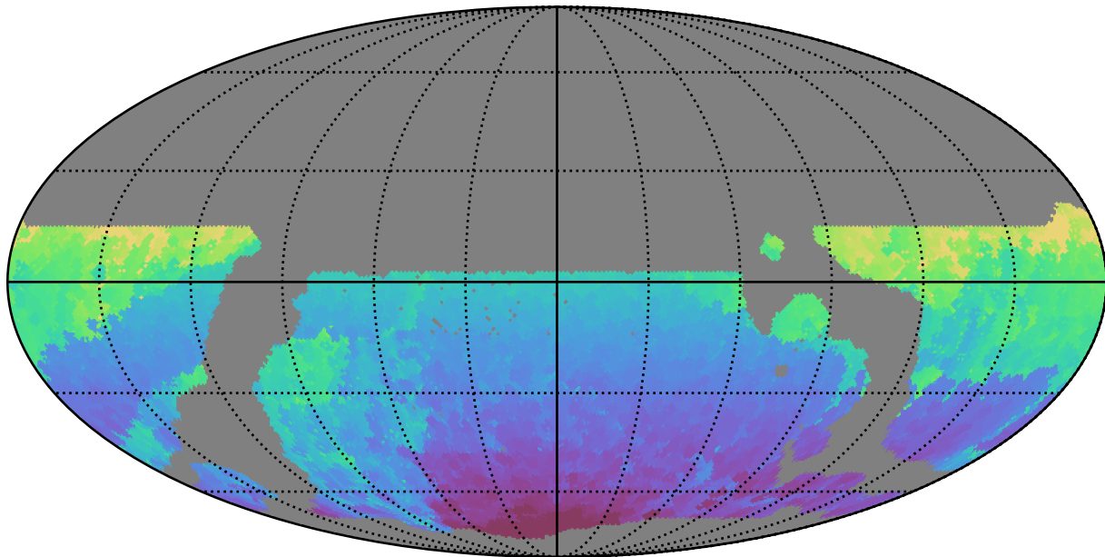
weather_cloudso35v3.4_10yrs WFD r band: Min HA
