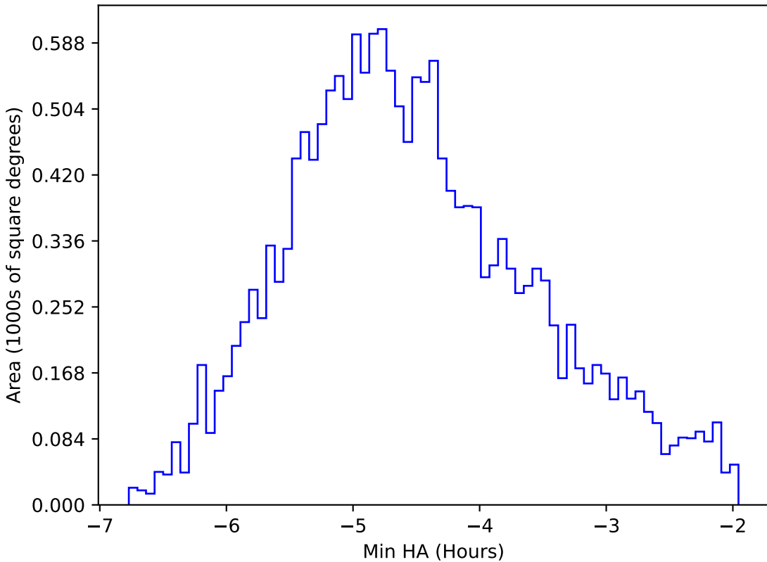
weather_cloudso35v3.4_10yrs WFD r band: Min HA
