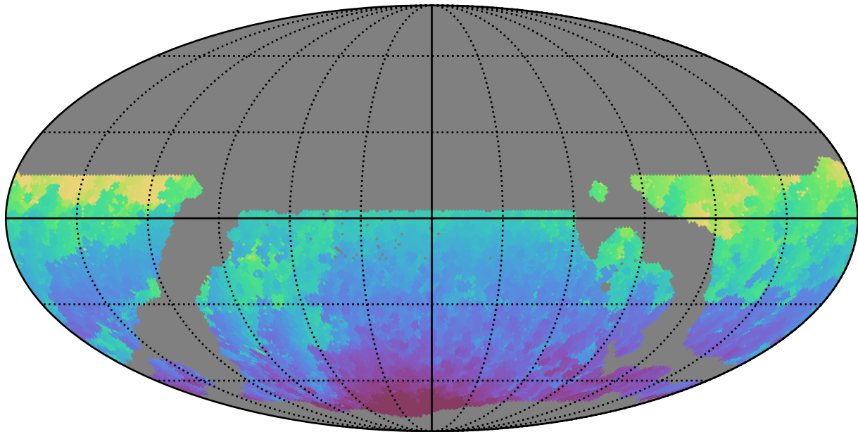
weather_cloudso35v3.4_10yrs WFD i band: Min HA
