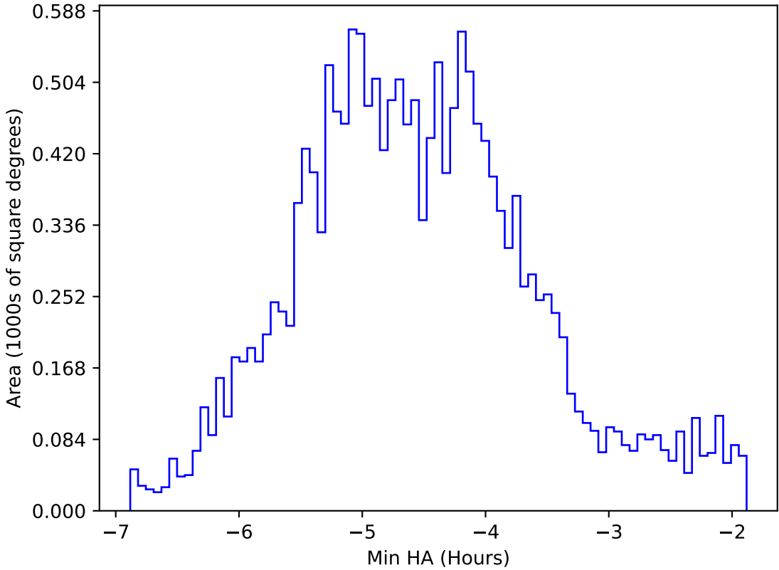
weather_cloudso35v3.4_10yrs WFD i band: Min HA
