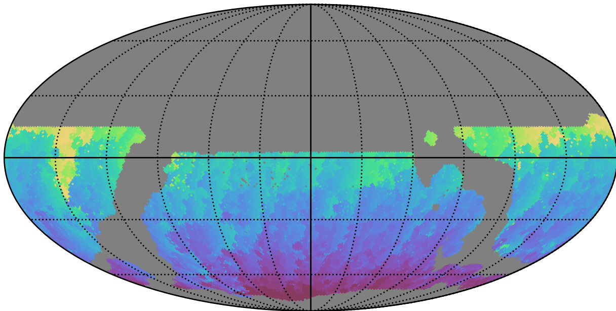
weather_cloudso35v3.4_10yrs WFD g band: Min HA
