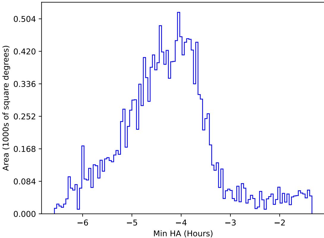
weather_cloudso35v3.4_10yrs WFD g band: Min HA
