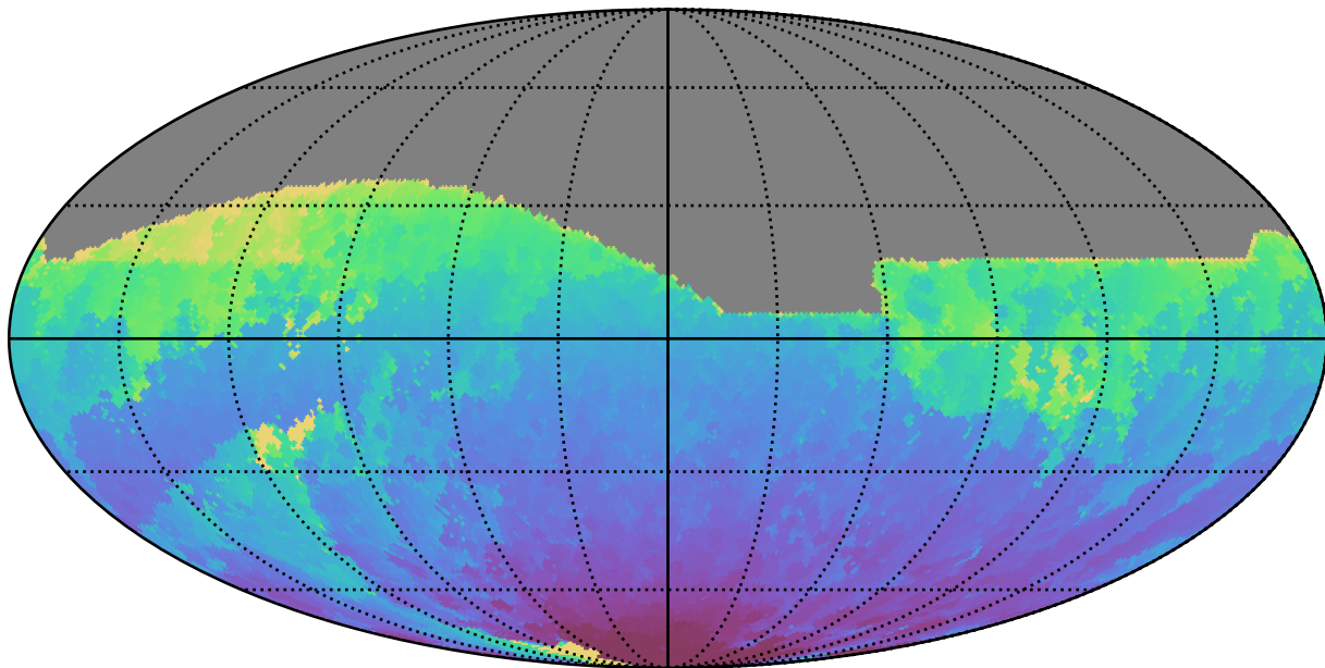
weather_cloudso35v3.4_10yrs All sky z band: Min HA
