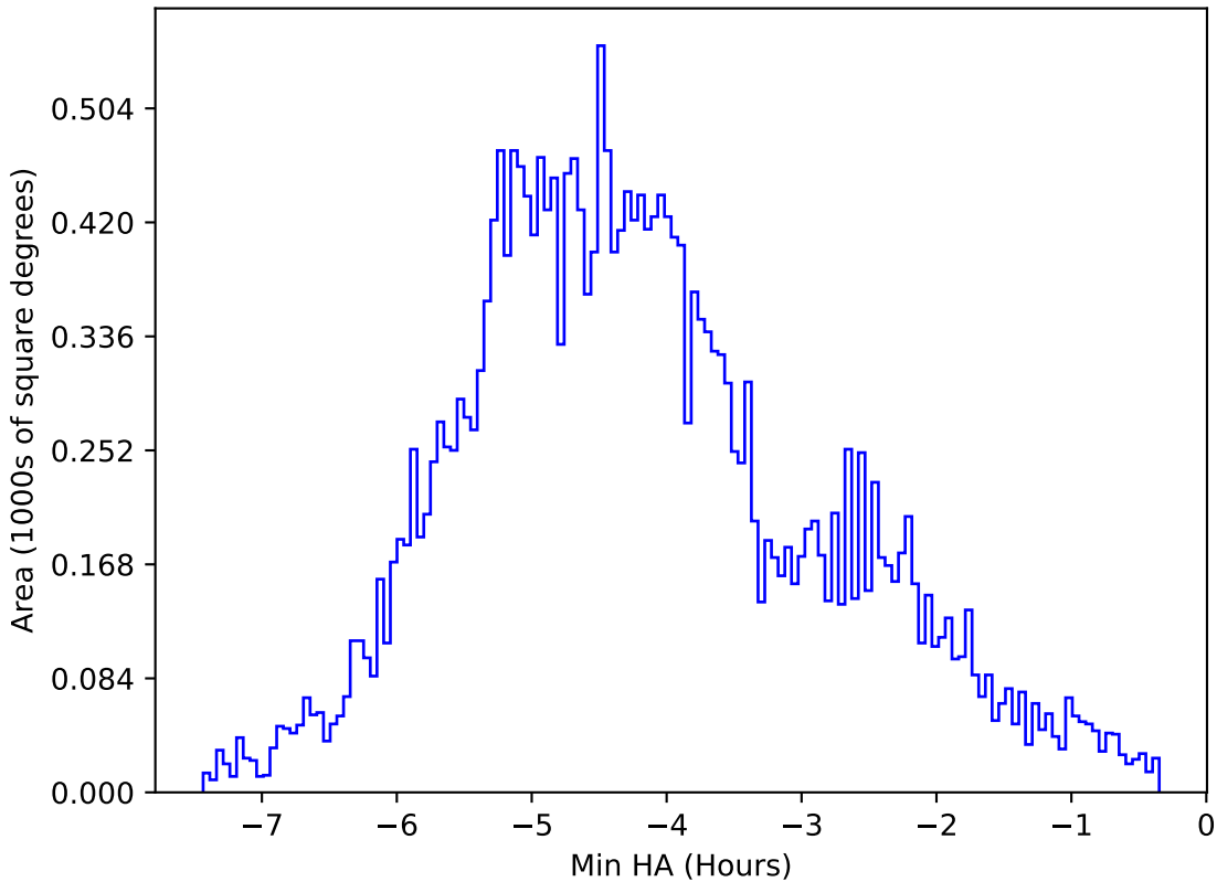
weather_cloudso35v3.4_10yrs All sky z band: Min HA
