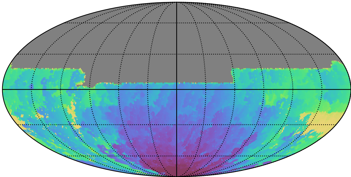
weather_cloudso35v3.4_10yrs All sky u band: Min HA
